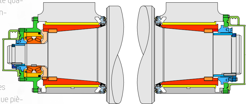
Vue en coupe avec les composants principaux
